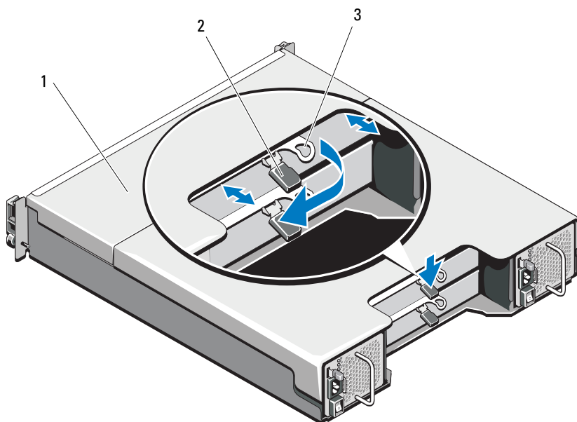
图 16-8. 卸下和安装 RAID 控制器模块
